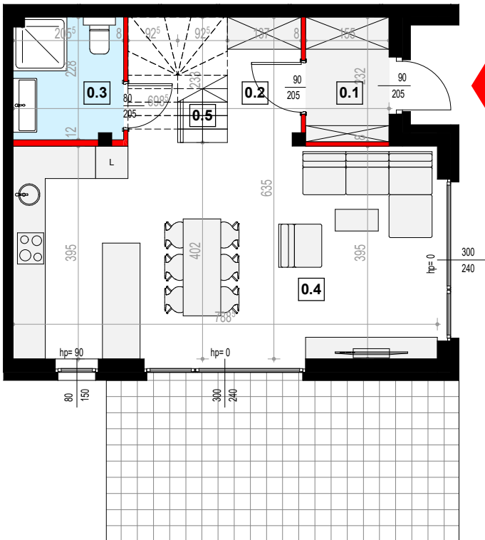
rzut parteru
